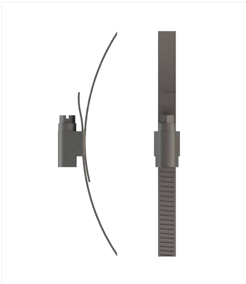
Schneckengewindegewinde nach DIN 3017 / Worm thread clamps DIN 3017
